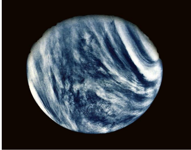
Image - Vénus par Mariner 10 mission Credit: NASA
